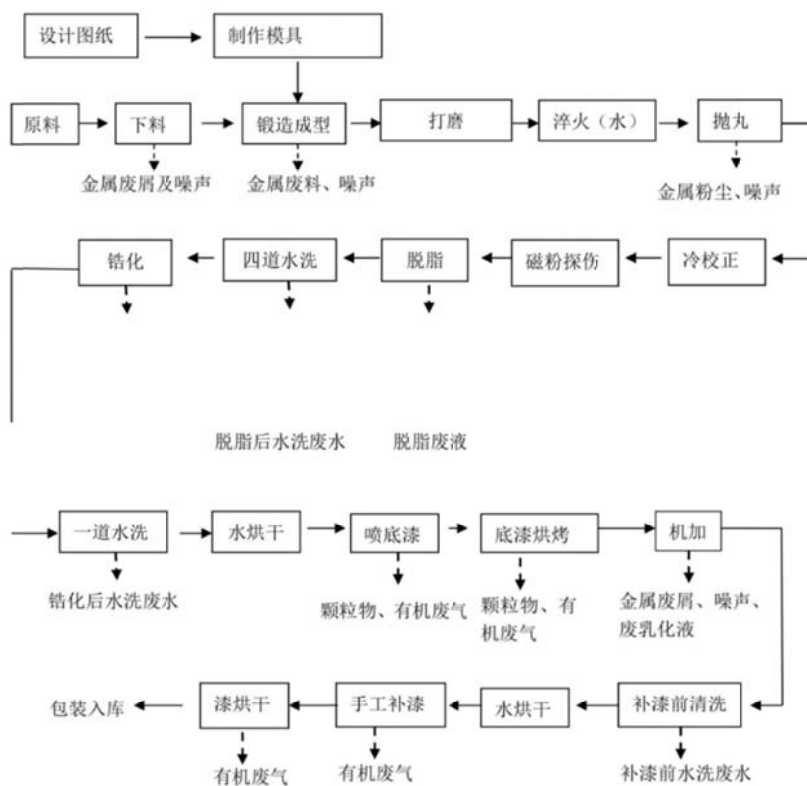
全厂生产工艺流程及产污节点图
